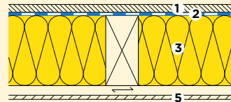
Variante 1 : Assainissement par le dessus et le dessous
