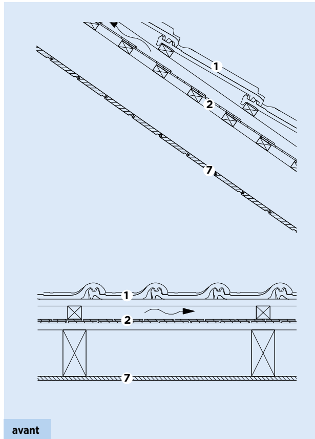
Variante SIA 380/1 avec bardeaux et isolation entre bardeaux
