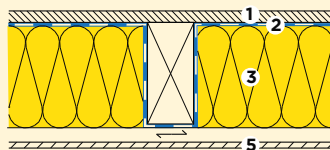
Variante 2 : Assainissement par le dessous
