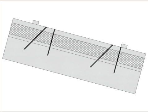
System-Verschraubung*: 30° und 90° zur Sparrenachse, kontinuierliche Verschraubung
