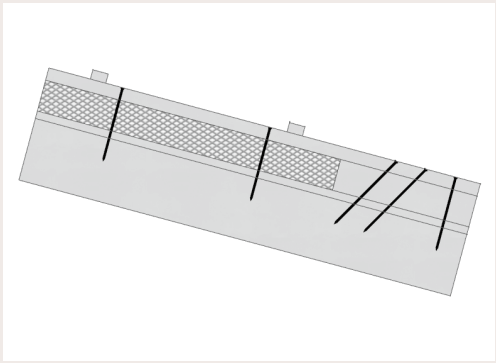
System-Verschraubung*: 90° zur Sparrenachse, mit Schrägschrauben im Aufschiebling
