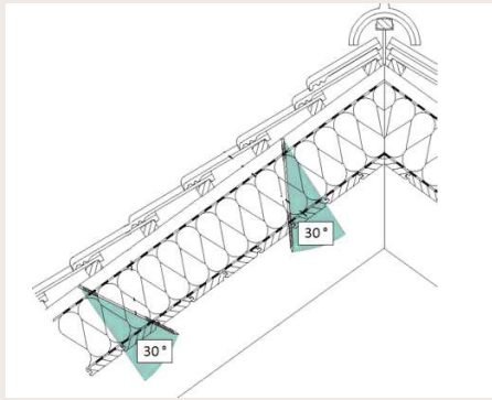
System-Verschraubung*: 30° zur Sparrenachse, abwechselnd (Flumserdach)
